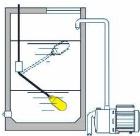
Sterowanie napełnianiem zbiornika
