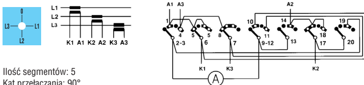
97 - Przelączniki amperometry bezpośredni odczytu prądu lub przez przekładniki prądowe
