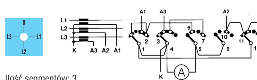
98 - Przelączniki amperometry do odczytu L1-L2-L3 przez 3 przekładniki prądowe
