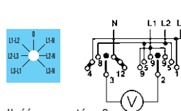
66 - Przelączniki woltometry, napięcia fazowe i międzyfazowe
