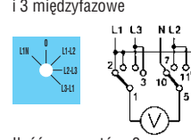
60 - Przelączniki woltometry, 1 napięcia fazowe i 3 międzyfazowe
